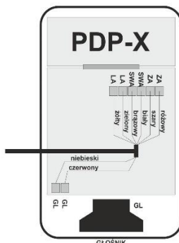
SCHEMAT PODŁĄCZENIA
